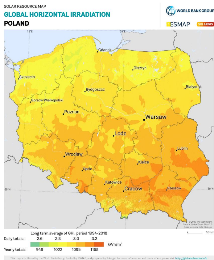
Mapa 5 - Mapa nasłonecznienia poziomej powierzchni Polski.
